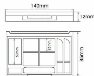
YH-E535C SIZE:L140*W85*H12mm
