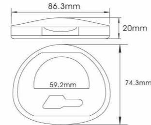
YH-E567B SIZE:L86.3*W74.3*H20mm
