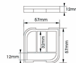
YH-E554E SIZE:L57*W57*H12mm
