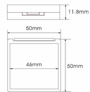
YH-E512A SIZE:W50*H11.8mm
