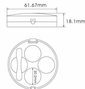
YH-E570B SIZE:W61.67*H18.1mm
