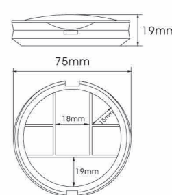
YH-E524C SIZE:W75*H19mm
