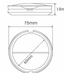
YH-E524B SIZE:W75*H19mm
