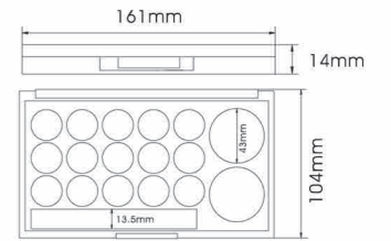
YH-E572C SIZE:L161*W104*H14mm
