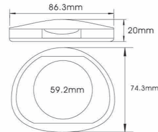
YH-E567A SIZE:L86.3*W74.3*H20mm
