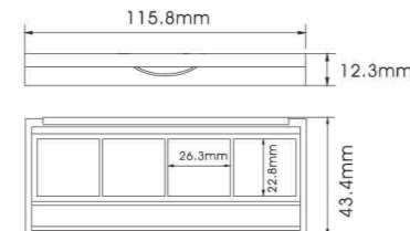
YH-E551C SIZE:L115.8*W43.4*H12.3mm
