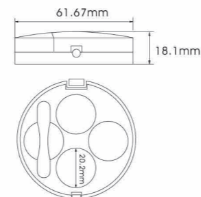
YH-E570 SIZE:W61.67*H18.1mm
