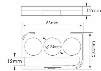
YH-E557A SIZE:L83*W50.5*H12mm
