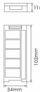
YH-E578A SIZE:L34*W102*H11mm
