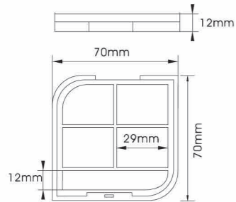
YH-E555G SIZE:L70*W70*H12mm
