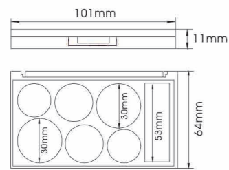
YH-E284D SIZE:L101*W64*H11mm
