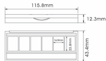
YH-E551E SIZE:L115.8*W43.4*H12.3mm
