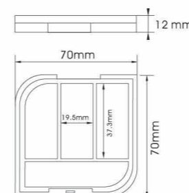
YH-E555E SIZE:L70*W70*H12mm
