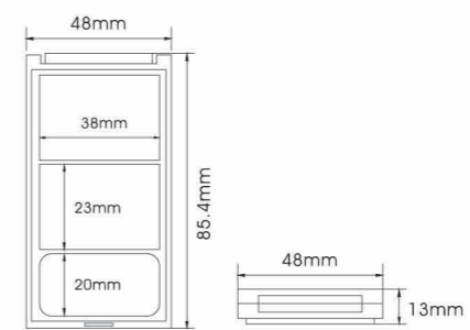
YH-E516A SIZE:L48*W85.4*H13mm
