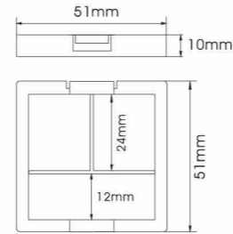
YH-E519C SIZE:W51*H10mm
