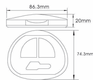
YH-E567C SIZE:L86.3*W74.3*H20mm
