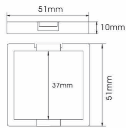
YH-E519A SIZE:W51*H10mm
