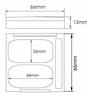
YH-E515E SIZE:W66*H12mm
