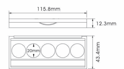
YH-E551A SIZE:L115.8*W43.4*H12.3mm
