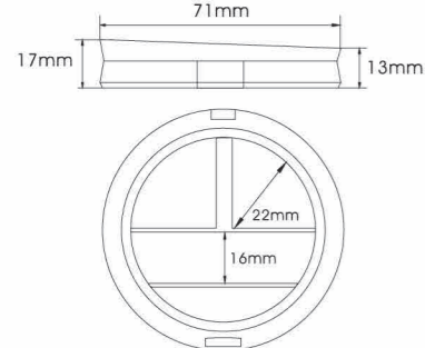
YH-E510 SIZE:W71*H17mm
