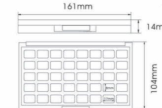
YH-E572A SIZE:L161*W104*H14mm
