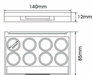
YH-E535A SIZE:L140*W85*H12mm
