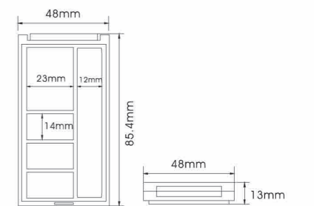
YH-E516B SIZE:L48*W85.4*H13mm
