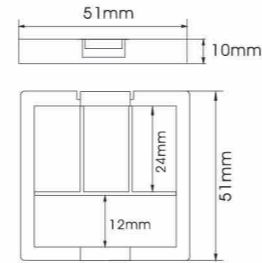
YH-E519D SIZE:W51*H10mm
