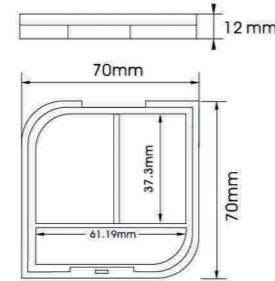
YH-E555C SIZE:L70*W70*H12mm
