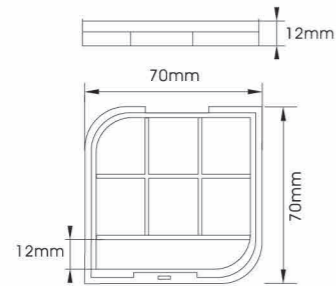
YH-E555H SIZE:L70*W70*H12mm
