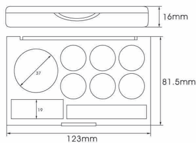
YH-E577 SIZE:L123*W81.5*H16mm
