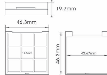
YH-E566 SIZE:L46.3*W46.3*H19.7mm
