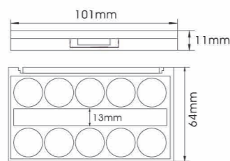
YH-E284K SIZE:L101*W64*H11mm
