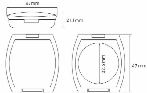
YH-E581 SIZE:W47*H21.1mm
