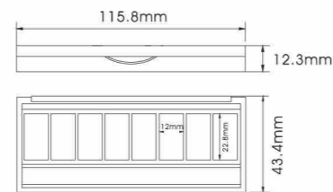
YH-E551F SIZE:L115.8*W43.4*H12.3mm
