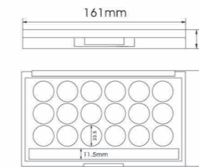
YH-E572E SIZE:L161*W104*H14mm
