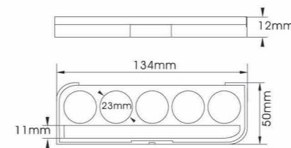
YH-E556B SIZE:L134*W50*H12mm
