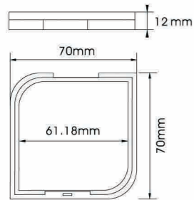
YH-E555A SIZE:L70*W70*H12mm
