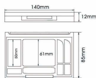
YH-E535B SIZE:L140*W85*H12mm
