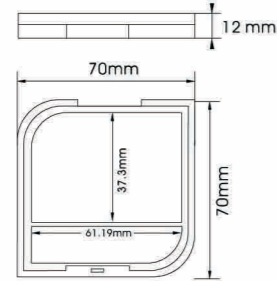
YH-E555B SIZE:L70*W70*H12mm
