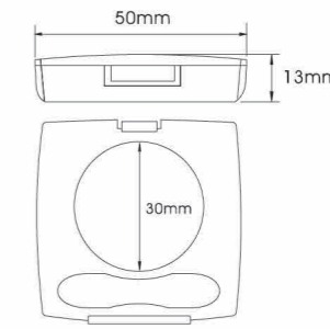
YH-E539A SIZE:W50*H13mm
