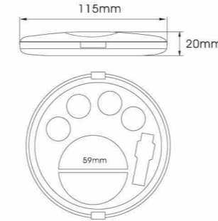
YH-E571 SIZE:L115*W115*H20mm
