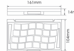
YH-E572B SIZE:L161*W104*H14mm
