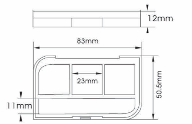
YH-E557B SIZE:L83*W50.5*H12mm
