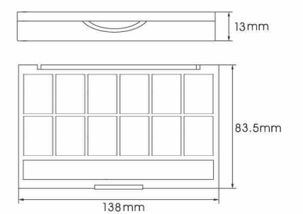
YH-E583 SIZE:L138*W83.5*H13mm
