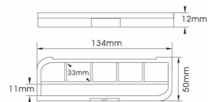
YH-E556A SIZE:L134*W50*H12mm
